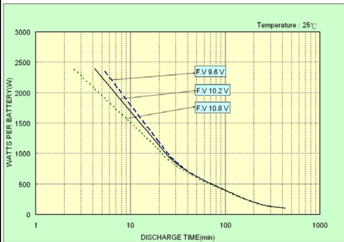
4.放電負載與放電時間的關係 (Discharge Characteristics of Constant Load)
